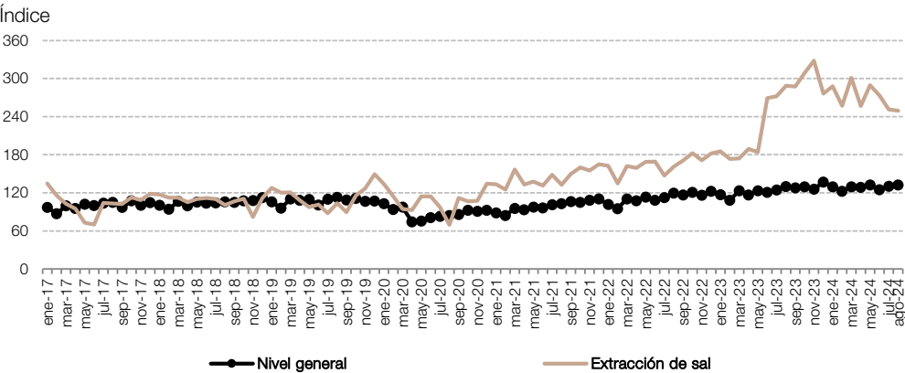
Gráfico 4.6.1 Extracción de sal respecto al Nivel general del IPI minero, en números índice. Enero 2017-agosto 2024
