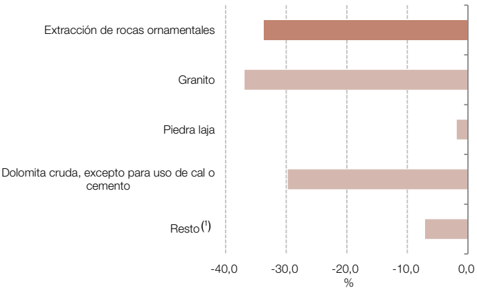
Gráfico 4.1.2 Extracción de rocas ornamentales, variación porcentual interanual. Agosto de 2024
