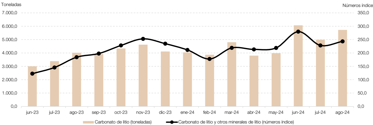
Gráfico 8. Carbonato de litio y otros minerales de litio, en toneladas y números índice. Junio 2023-agosto 2024
