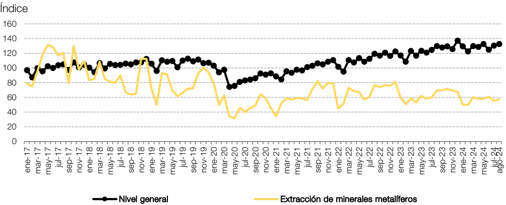
Gráfico 3.1 Extracción de minerales metalíferos respecto al Nivel general del IPI minero, en números índice. Enero 2017-agosto 2024
