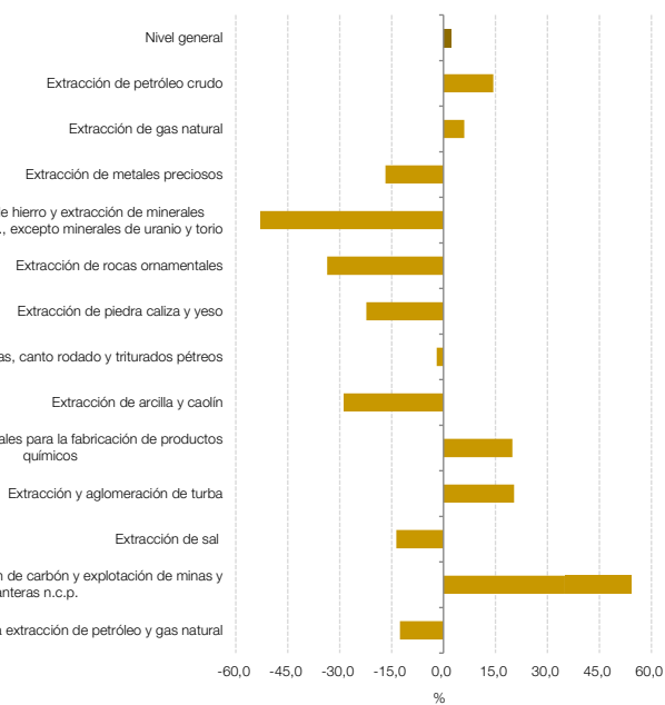
Gráfico 5.1 IPI minero Nivel general y subclases, variación porcentual interanual. Agosto de 2024
