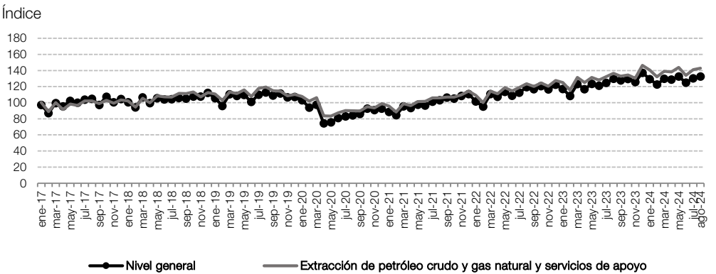
Gráfico 2.1 Extracción de petróleo crudo y gas natural y servicios de apoyo respecto al Nivel general del IPI minero, en números índice. Enero 2017-agosto 2024
