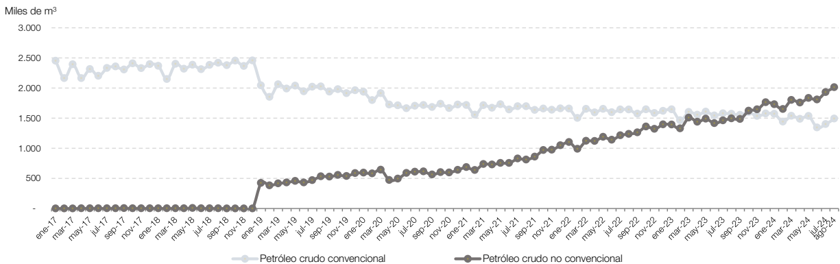
Gráfico 6.2 Extracción de petróleo crudo convencional y no convencional, en miles de m³. Enero 2017-agosto 2024
