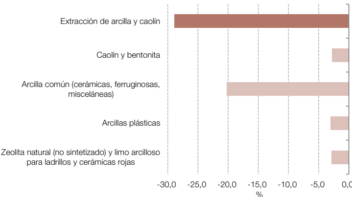
Gráfico 4.4.3 Extracción de arcilla y caolín, incidencias. Agosto de 2024
