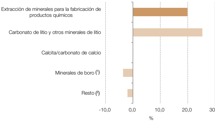
Gráfico 4.5.3 Extracción de minerales para la fabricación de productos químicos, incidencias. Agosto de 2024
