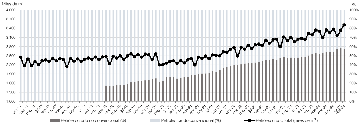
Gráfico 6.1 Extracción de petróleo crudo convencional y no convencional, en miles de m³ y estructura porcentual. Enero 2017-agosto 2024
