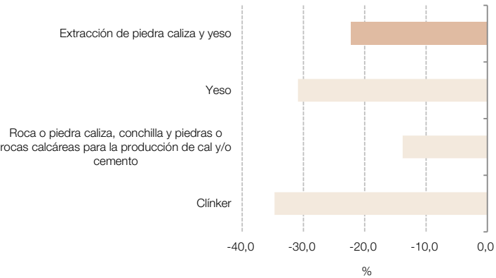
Gráfico 4.2.2 Extracción de piedra caliza y yeso, variación porcentual interanual. Agosto de 2024
