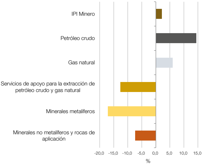
Gráfico 1.2 IPI minero Nivel general y categorías, variación porcentual interanual. Agosto de 2024
