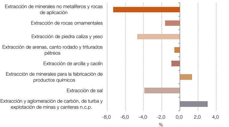
Gráfico 4.3 Minerales no metalíferos y rocas de aplicación, incidencias. Agosto de 2024
