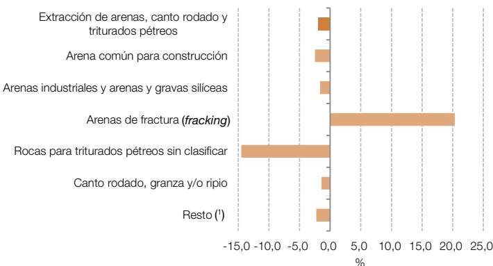
Gráfico 4.3.3 Extracción de arenas, canto rodado y triturados pétreos, incidencias. Agosto de 2024
