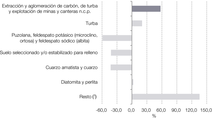
Gráfico 4.7.2 Carbón, turba y explotación de minas y canteras n.c.p., variación porcentual interanual. Agosto de 2024
