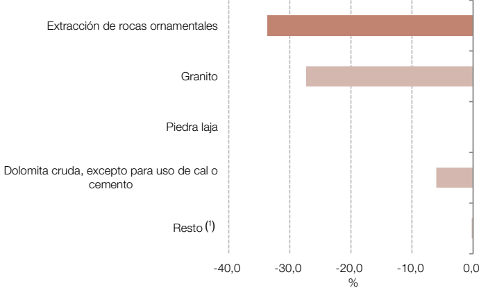
Gráfico 4.1.3 Extracción de rocas ornamentales, incidencias. Agosto de 2024
