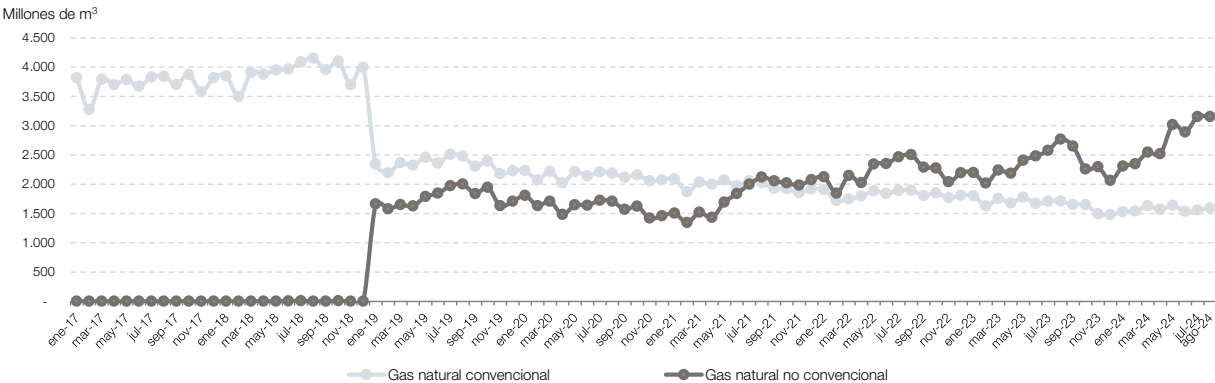
Gráfico 7.2 Extracción de gas natural convencional y no convencional, en millones de m³. Enero 2017-agosto 2024
