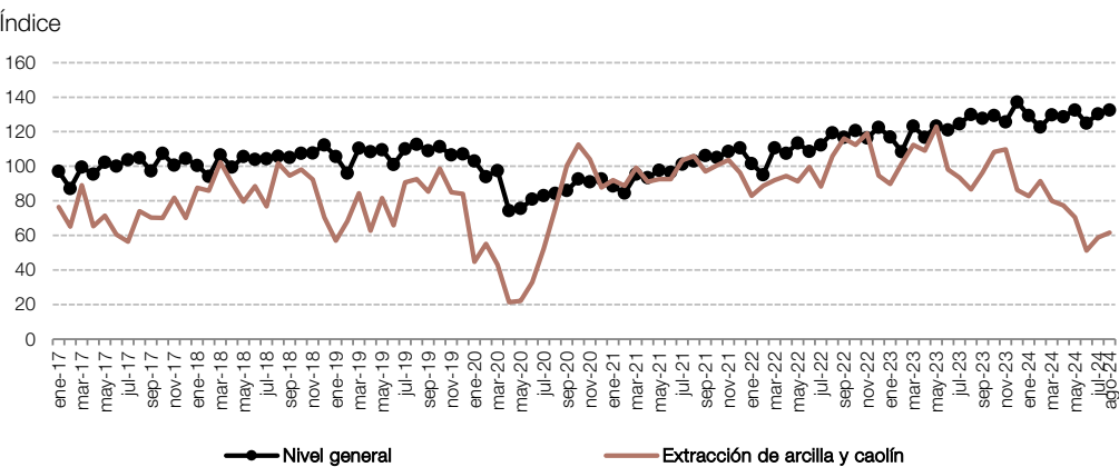
Gráfico 4.4.1 Extracción de arcilla y caolín respecto al Nivel general del IPI minero, en números índice. Enero 2017-agosto 2024
