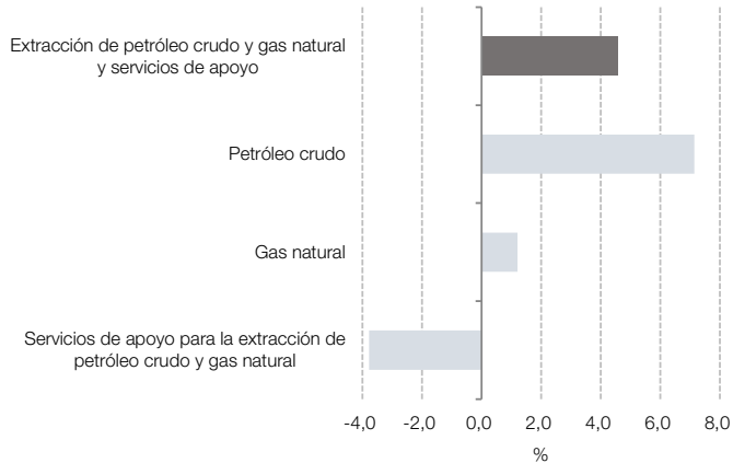
Gráfico 2.3 Petróleo crudo, gas natural y servicios de apoyo, incidencias. Agosto de 2024
