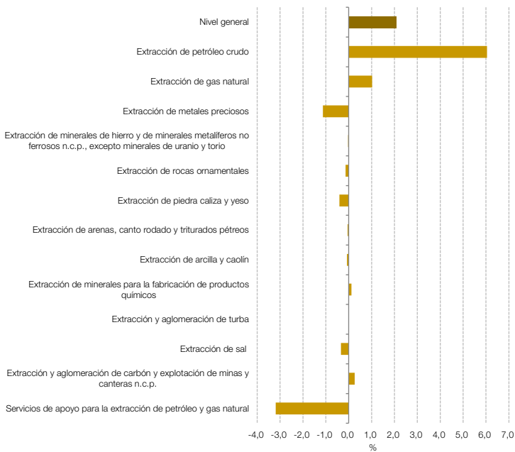
Gráfico 5.2 IPI minero Nivel general y subclases, incidencias. Agosto de 2024
