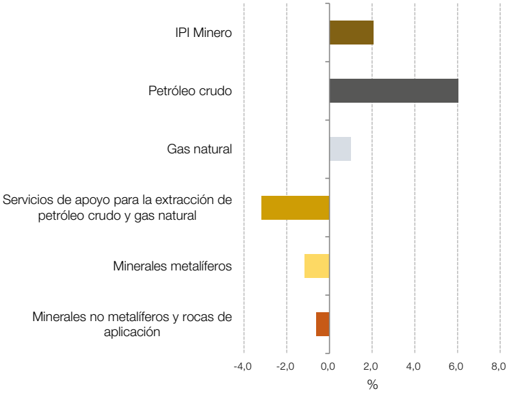
Gráfico 1.3 IPI minero Nivel general y categorías, incidencias. Agosto de 2024
