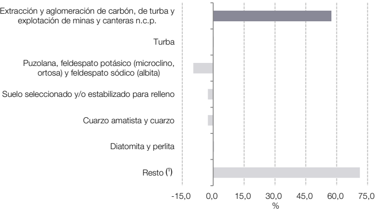
Gráfico 4.7.3 Carbón, turba y explotación de minas y canteras n.c.p., incidencias. Agosto de 2024
