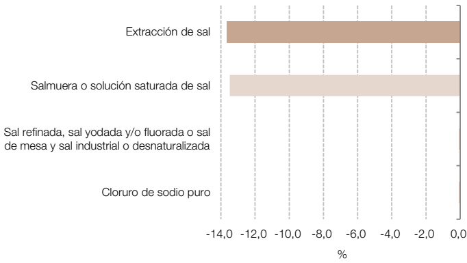
Gráfico 4.6.3 Extracción de sal, incidencias. Agosto de 2024
