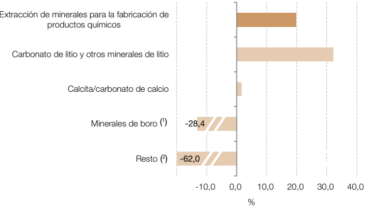
Gráfico 4.5.2 Extracción de minerales para la fabricación de productos químicos, variación porcentual interanual. Agosto de 2024
