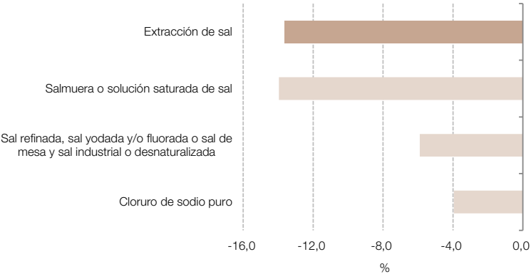
Gráfico 4.6.2 Extracción de sal, variación porcentual interanual. Agosto de 2024
