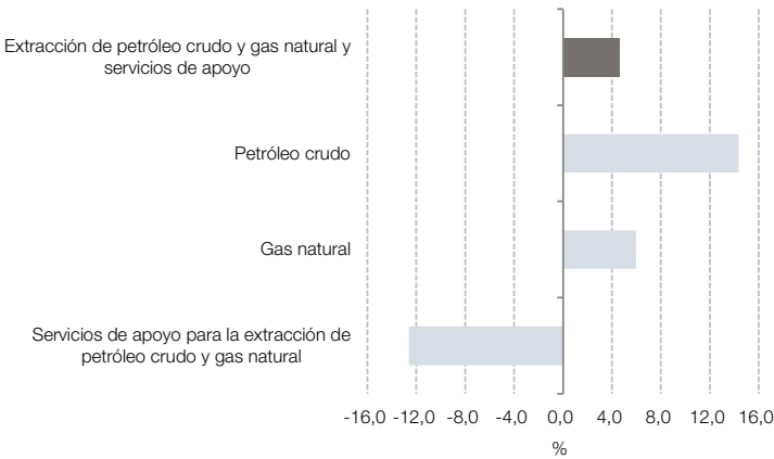
Gráfico 2.2 Petróleo crudo, gas natural y servicios de apoyo, variación porcentual interanual. Agosto de 2024
