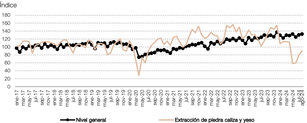
Gráfico 4.2.1 Extracción de piedra caliza y yeso respecto al Nivel general del IPI minero, en números índice. Enero 2017-agosto 2024
