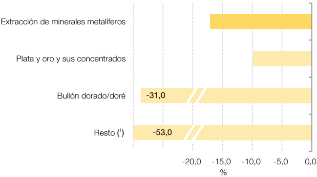
Gráfico 3.2 Extracción de minerales metalíferos, variación porcentual interanual. Agosto de 2024
