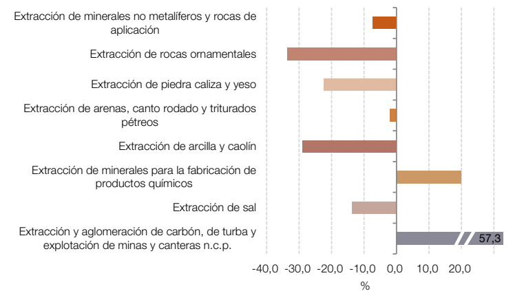
Gráfico 4.2 Minerales no metalíferos y rocas de aplicación, variación porcentual interanual. Agosto de 2024
