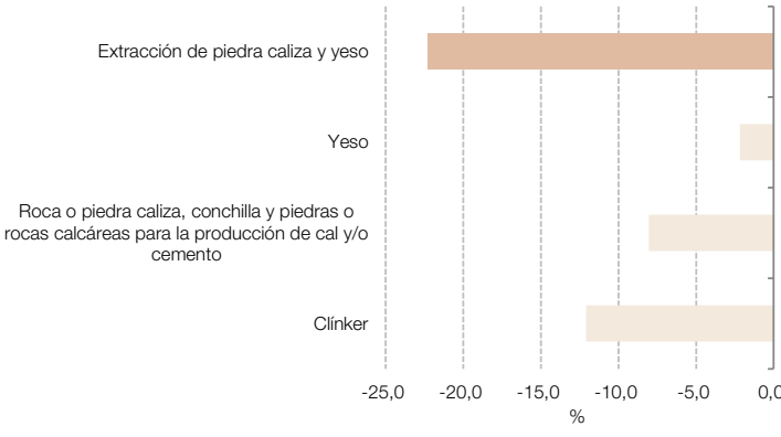
Gráfico 4.2.3 Extracción de piedra caliza y yeso, incidencias. Agosto de 2024
