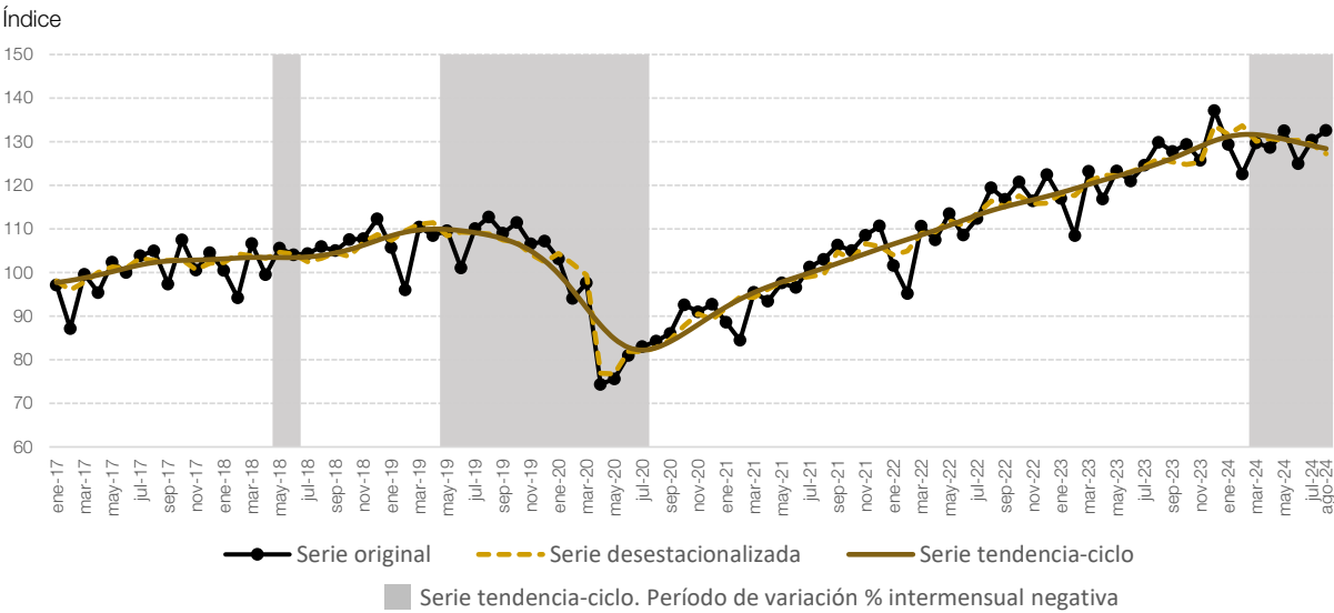
Gráfico 1.1 IPI minero Nivel general. Serie original, desestacionalizada y tendencia-ciclo, base 2016=100, en números índice. Enero 2017-agosto 2024
