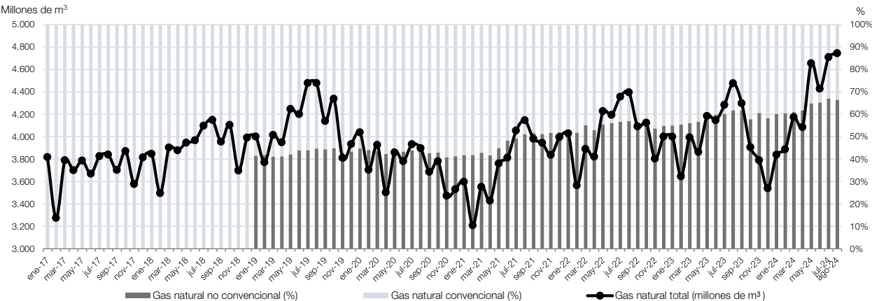
Gráfico 7.1 Extracción de gas natural convencional y no convencional, en millones de m³ y estructura porcentual. Enero 2017-agosto 2024
