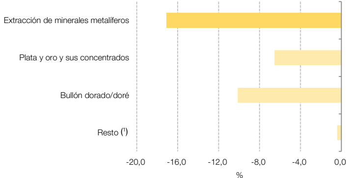
Gráfico 3.3 Extracción de minerales metalíferos, incidencias. Agosto de 2024
