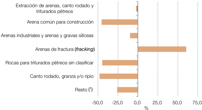
Gráfico 4.3.2 Extracción de arenas, canto rodado y triturados pétreos, variación porcentual interanual. Agosto de 2024
