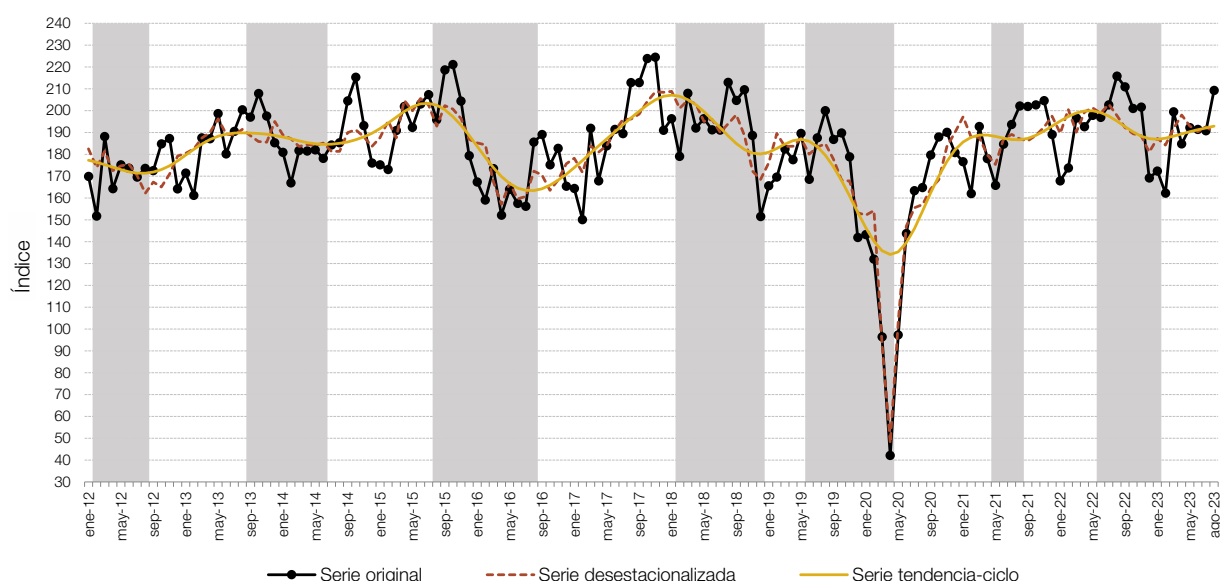
Gráfico 1. Indicador sintético de la actividad de la construcción (ISAC). Serie original, desestacionalizada y tendencia-ciclo, base 2004=100, en números índice. Enero 2012-agosto 2023
