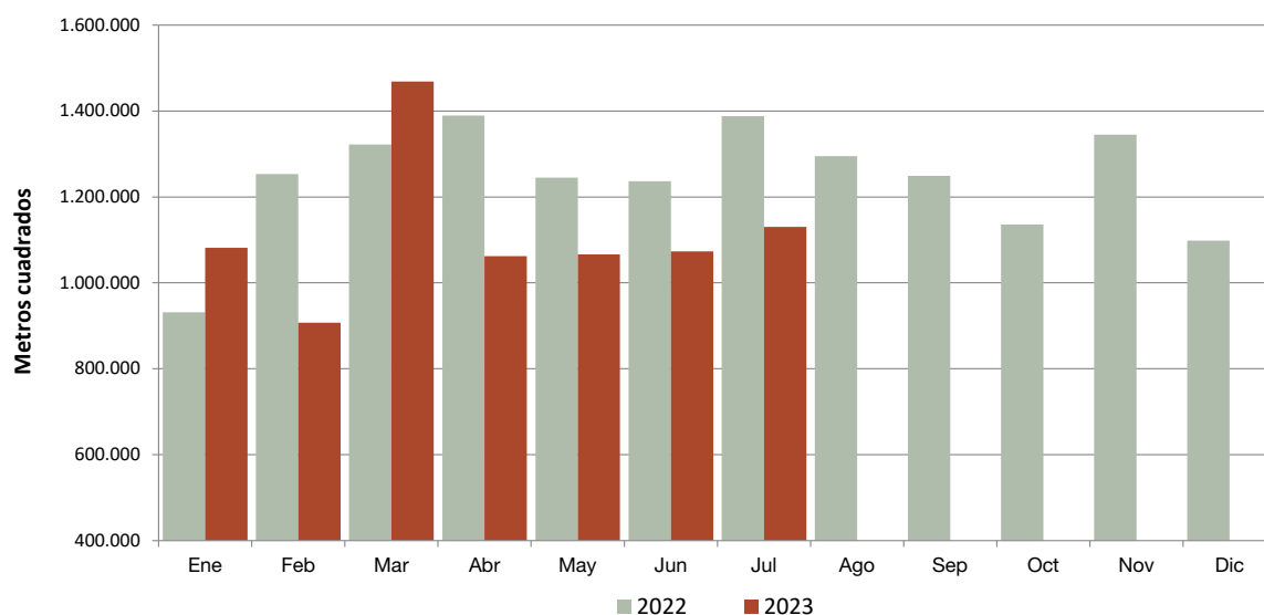
Gráfico 4.1 Superficie autorizada por los permisos de edificación, en metros cuadrados. Enero 2022-julio 2023
