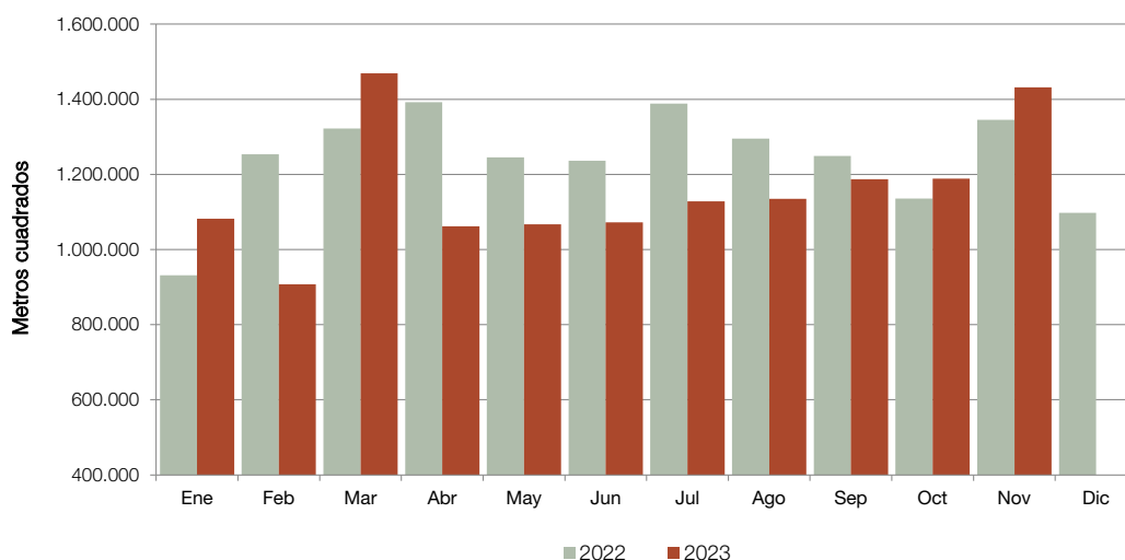
Gráfico 4.1 Superficie autorizada por los permisos de edificación, en metros cuadrados. Enero 2022-noviembre 2023
