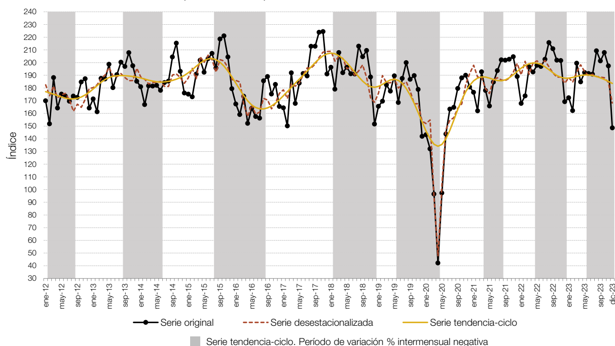
Gráfico 1. Indicador sintético de la actividad de la construcción (ISAC). Serie original, desestacionalizada y tendencia-ciclo, base 2004=100, en números índice. Enero 2012-diciembre 2023
